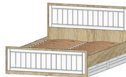
КРОВАТЬ 2х сп. 1400 1432(Ш) x 2048(Г) x 909(В) мм (ортопедическое основание)
