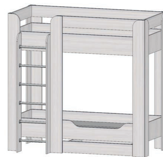
КРОВАТЬ 2x ЯРУСНАЯ 1924(Ш) x 1000(Г) x 1830(В) мм универсальная сборка, спальное место 1860x800 мм - 2 шт, ширина лестницы 430 мм
