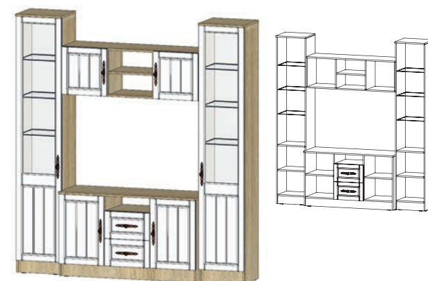
ЦЕНТРАЛЬНАЯ СЕКЦИЯ 2000(Ш) x 425(Г) x 2154(В) мм
