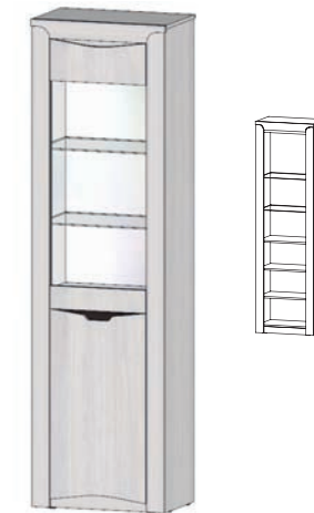
ПЕНАЛ СО СТЕКЛОМ 600(Ш) x 380(Г) x 2105(В) мм
