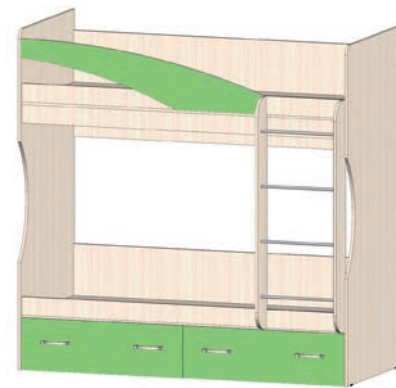
КРОВАТЬ 2х ЯРУСНАЯ 1892(Ш) x 982(Г) x 1855(В) мм размер под матрас 800x1860 мм универсальная сборка на любую сторону
